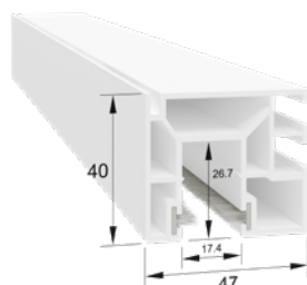
ROLL 960-2B mit zwei eingezogenen Bürstendichtungen
