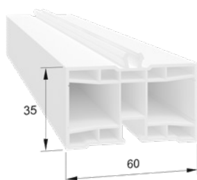
ARD960 Adapter für Doppelführungsschiene
