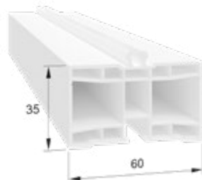
ARD960 Adapter für Doppelführungsschiene
