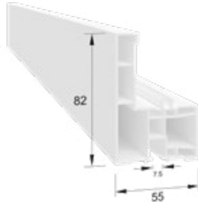
AR960 mit ROLL 960-2B zwingend notwendig für die Außenrevision ABR5021 (S, 74)
